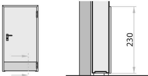
Zoccoli
