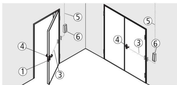
Schema componenti
