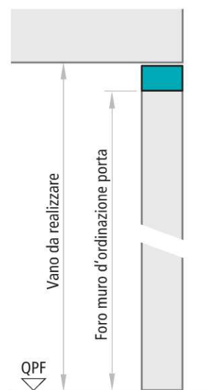
Sezione verticale
